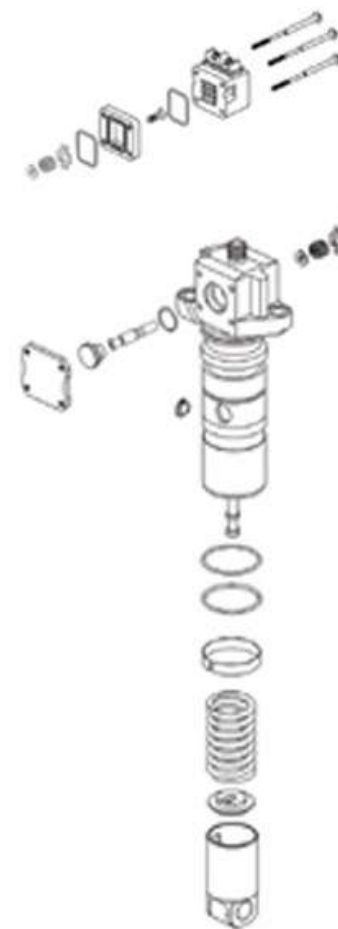
BOSCH® PLD/EUP 0414-755-...
